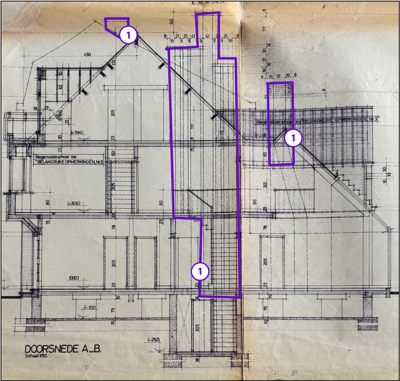
Legende van plan 1.7: DOORSNEE (2)
